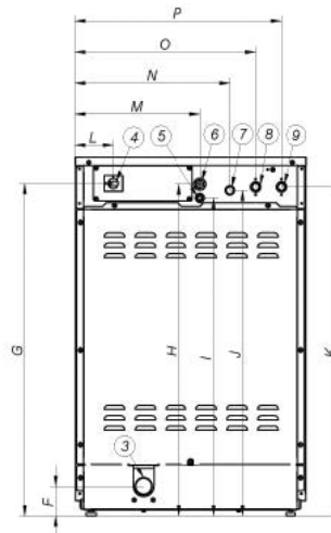
RÜCKANSICHT
