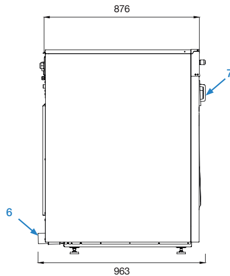
SEITENSICHT TWE10
