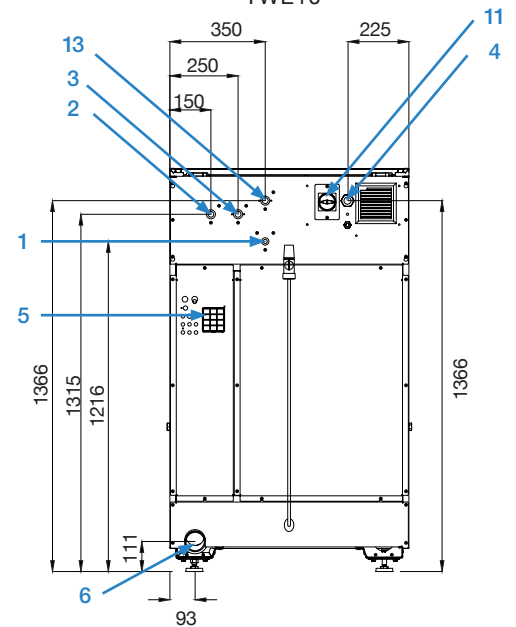
RÜCKANSICHT TWE10
